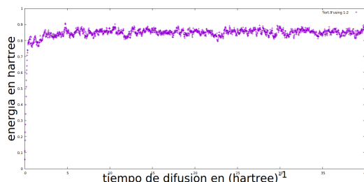
Figure 1: Energía fundamental con el potencial de Morse
