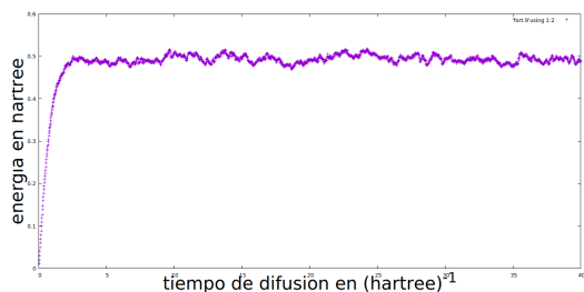
Figure 2: Energía fundamental para el Oscilador Armónico en una dimensión
