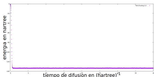
Figure 4: Potencial Polinomial de orden cuatro
