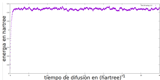
Figure 3: Energía fundamental del potencial Coseno Hiperbólico
